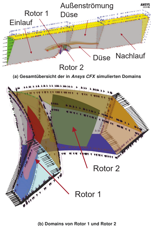
BILD 5. CFX Domains
