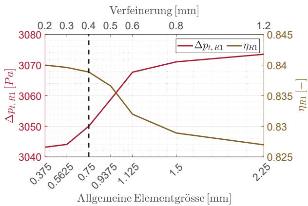
BILD 6. Abhängigkeit der Simulationsergebnisse von der allgemeinen Netzelementgröße (unten) und derer auf Verfeinerungen (oben)
