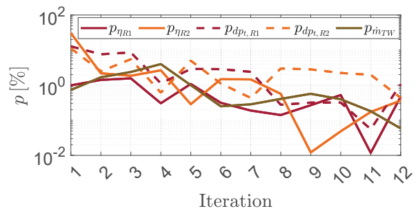
BILD 8. Iterative Entwicklung des Betrags der prozentualen Abweichungen p zwischen CDF-Ergebnissen und Eingangsparametern in die jeweilige Triebwerksauslegung
