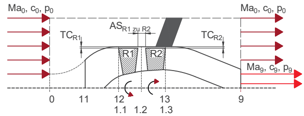
BILD 1. Schematische Darstellung des gegenläufigen, elektrischen Triebwerks unter Einbeziehung der Triebwerks- und Fanstufenebenen (obere und untere Zahlenreihe)
