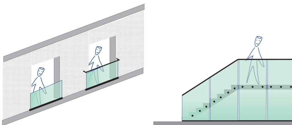
Bild 6 Beispiele für Fehlinterpretation von Kategorie B; Links: eingespannte Glasbrüstungen ohne Handlauf außerhalb der DIN 18008 und mit seitlich angeschlossener Handlauf Kategorie C; Rechts: Regelungslücke und denkbare Erweiterung der Kategorie B
