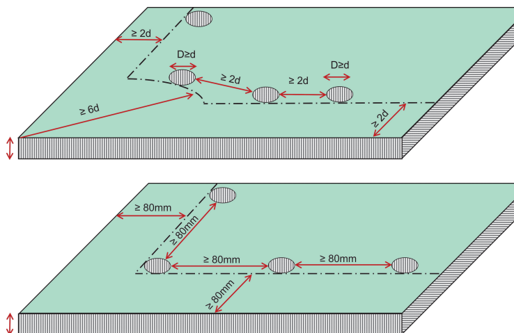
Bild 4 Bohrungsgeometrie nach Produktnorm (oben) und nach Bemessungsnorm DIN 18008 (unten), d = Plattendicke, D = Bohrungsdurchmesser
